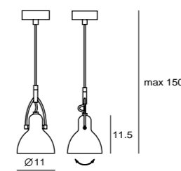
LAITO MINI P SQ-793MP E14 1 x Max 30W Halogen copper/ matt brass 紅銅/ 霧金 shade rotatable
